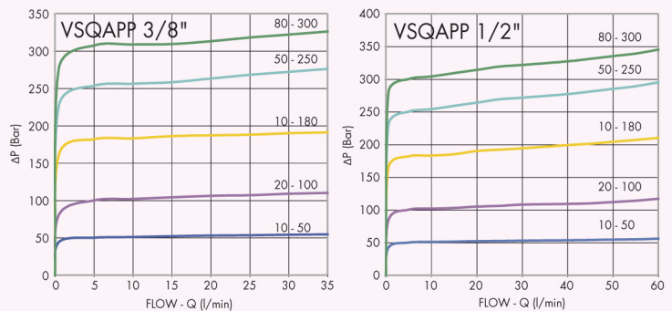
PRESSIONE/PORTATA PRESSURE/FLOW
