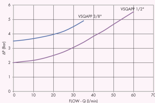
PERDITE DI CARICO PRESSURE DROPS CURVE
